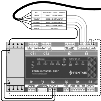
Figura 6: diagramma di cablaggio di ControlPro
