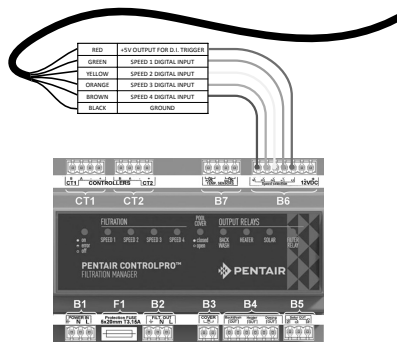
Abbildung 6: ControlPro+ Verdrahtungsdiagramm
