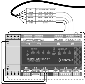
Abbildung 6: ControlPro Verdrahtungsdiagramm
