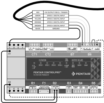
Figura 6: Diagrama de cableado ControlPro
