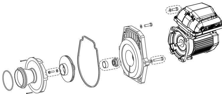
Motorgroep Whisperflo VS2
