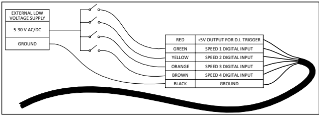
Figura 5: diagramma del cablaggio di alimentazione a bassa tensione
