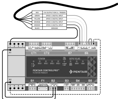
Figure 6 : Schéma de câblage ControlPro
