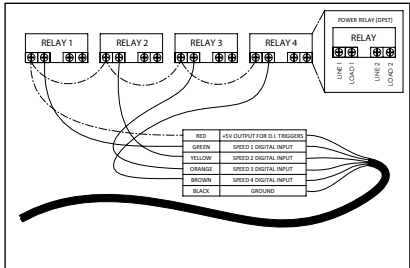
Abbildung 4: Verdrahtungsdiagramm der externen Steuerung
